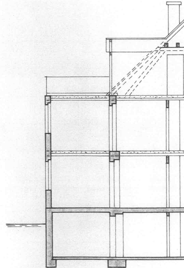
SCHNITT A-B
