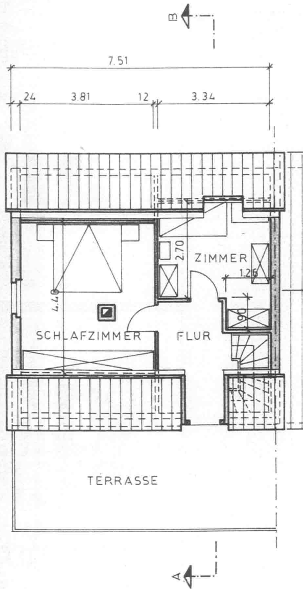
DACHGESCHOSS
